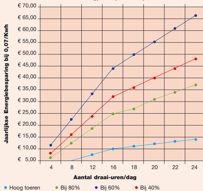
Besparingsgrafiek tussen normale AC ventilator (265 Watt) voorzien van toerenregeling d.m.v. fase aansnijding & de Holland Heater Low-Energy Fan (265 Watt)
