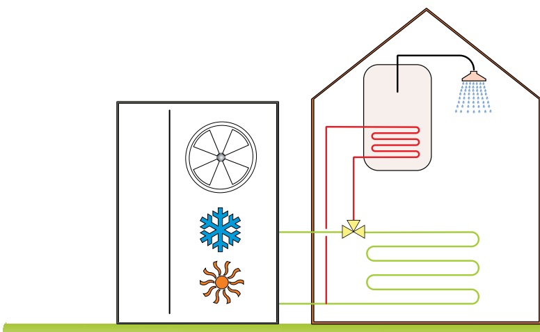
LZT 2 PIPES VERSION.
